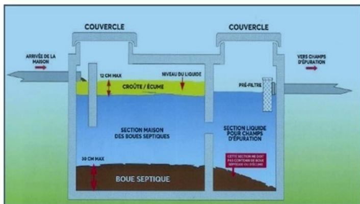
1 - Illustration des compartiments d'une fosse septique [gracieuseté d'Abi-Vac].
